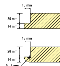
PROFIL HRANY
