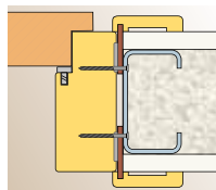
Montáž za pomoci šroubů do sádkartonové zdi
