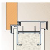
Montáž velké rohové zárubně do sádkartonových zdí.
