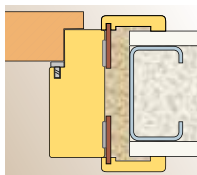
Montáž za pomoci pěny do sádkartonové zdi
